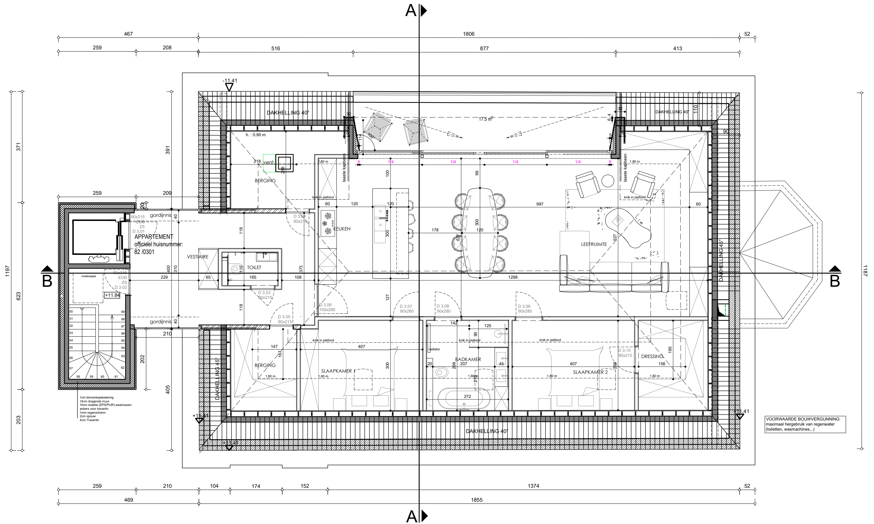
Grondplan Zolderverdieping (APP. 2) Nieuwe Toestand
